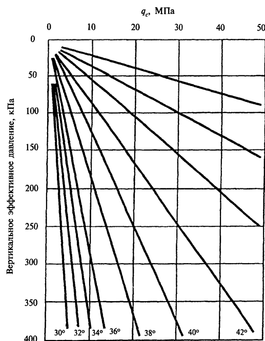
Рис. М2. Номограмма определения угла внутреннего трения песков по CPT (по Robertson and Campanella, 1983)
